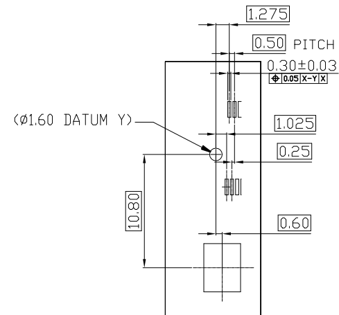
DETAIL:D SCALE 2:1
